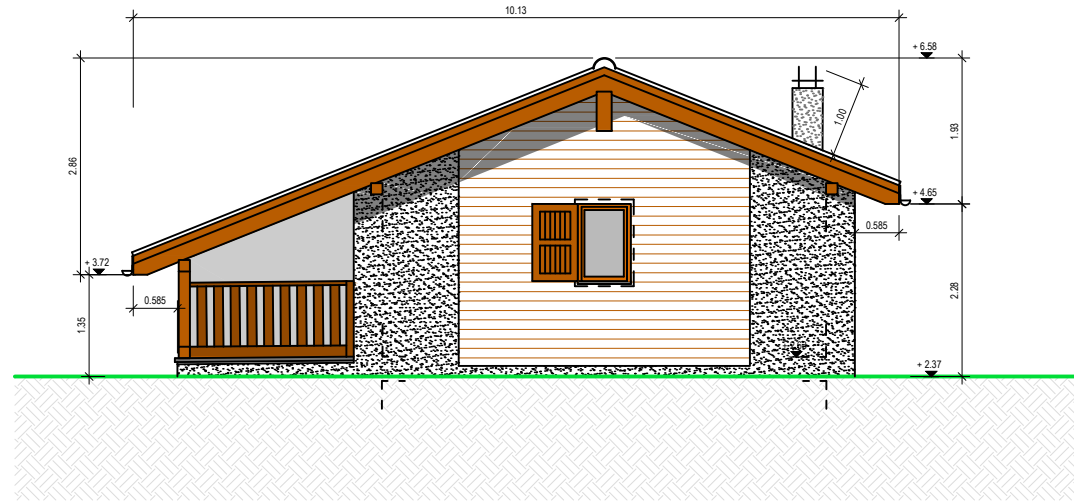
FACCIATA NORD
