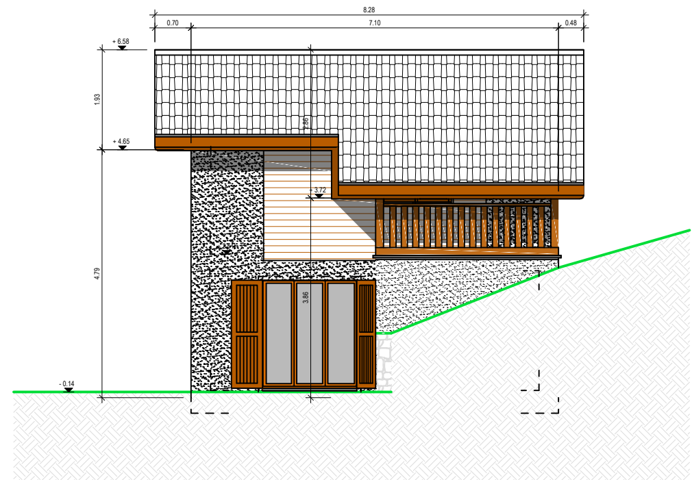
FACCIATA EST
