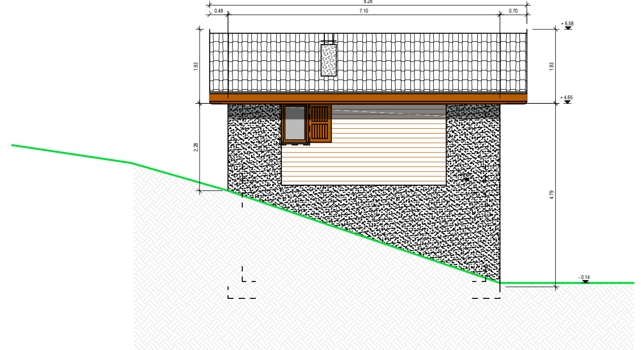
FACCIATA OVEST
